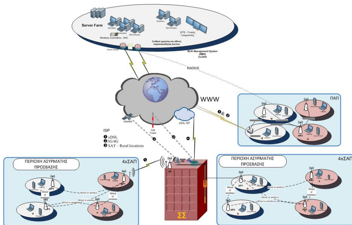
Σχήμα 4: Ενδεικτική Αρχιτεκτονική Κέντρου Διαχείρισης Δικτύου και επικοινωνία με ΠΑΠ
