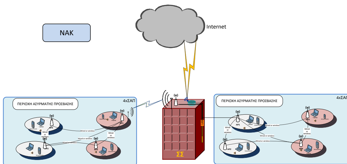
Σχήμα 3: Ενδεικτική Αρχιτεκτονική Νησίδας Ασύρματης Κάλυψης (Ενσύρματα ή Ασύρματα Σύνδεση ΠΑΠ με ΣΣ)
